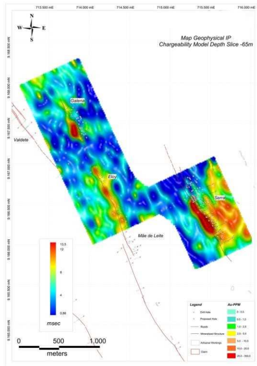
IP Survey
